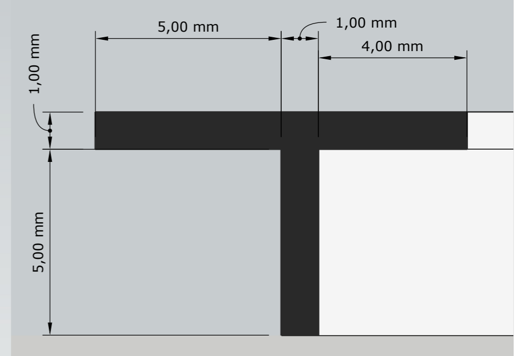
поперечное сечение профиля
