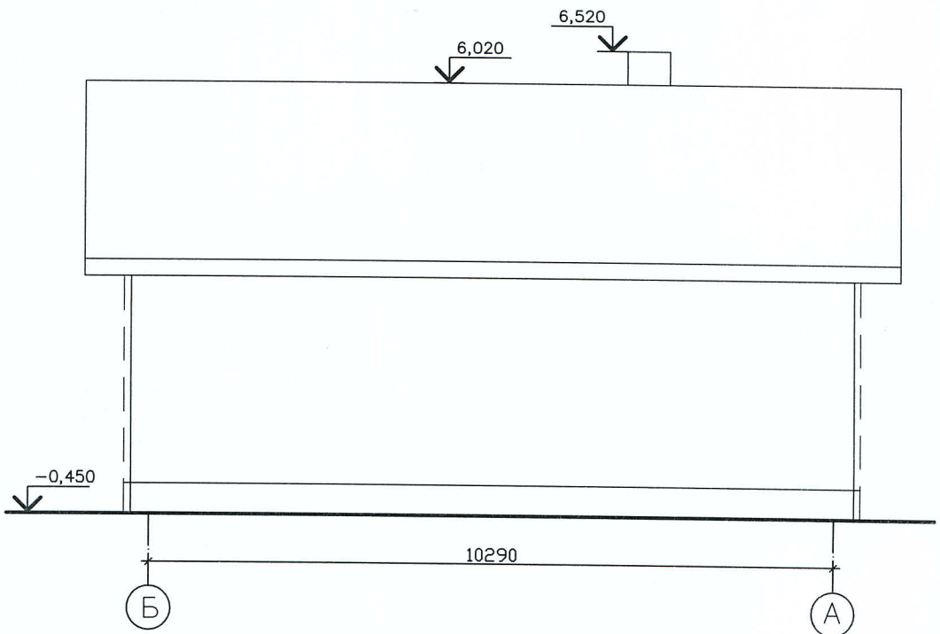
Фасад Б-А
