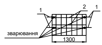
б-б (схема армування кладки)
