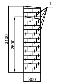
а-а (схема анкерування кладки)
