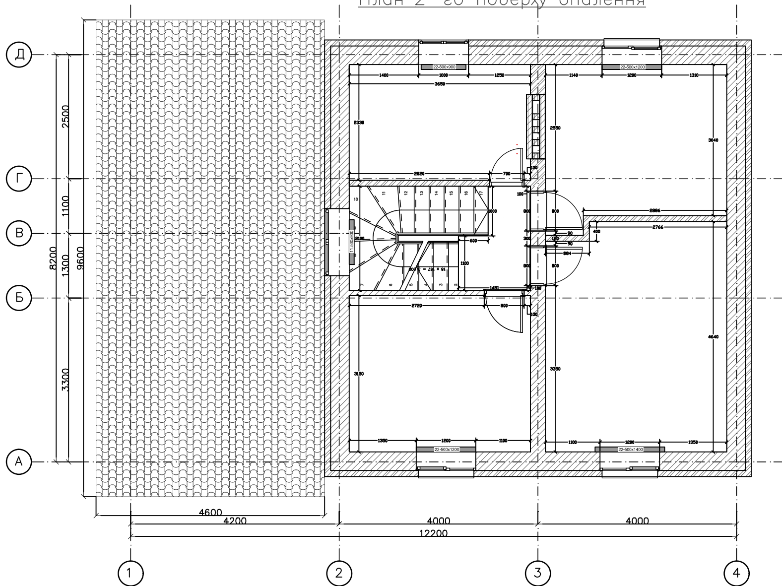
План 2-го поверху опалення
