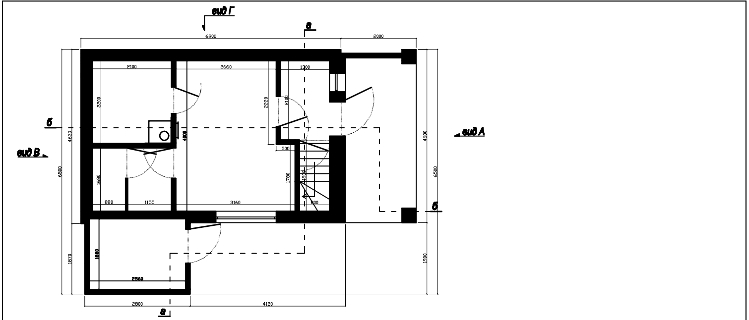
Баня - планировка - забаритные размеры
